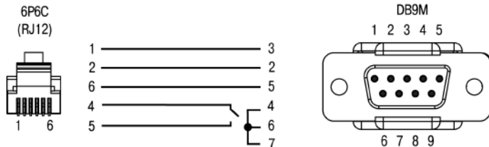
Рисунок В.2 - Схема кабеля KC3 для подключения модема к ПЛК154 по интерфейсу RS-232 Debug
